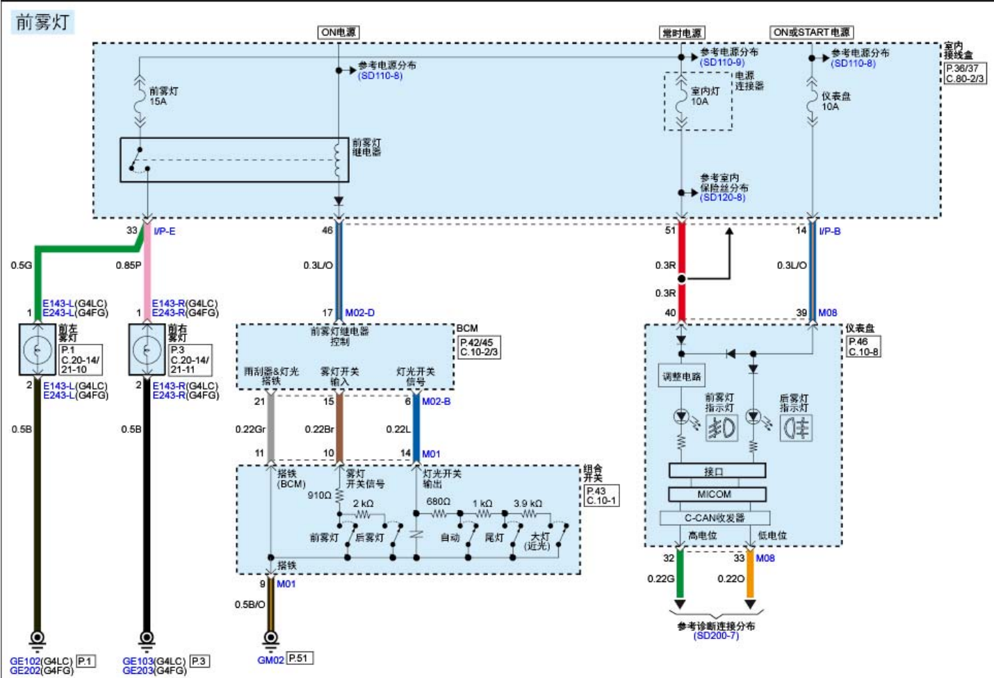
雾灯(1)
